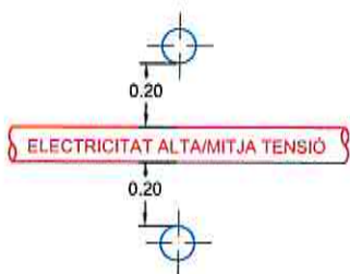
SECCIONS INSTAL·LACIONS SEPARACIONS VERTICALS A CREUAMENTS
