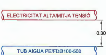
VISTA SUPERIOR INSTAL·LACIONS SEPARACIONS HORIZONTALS
