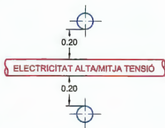
SECCIONS INSTAL·LACIONS SEPARACIONS VERTICALS A CREUAMENTS
