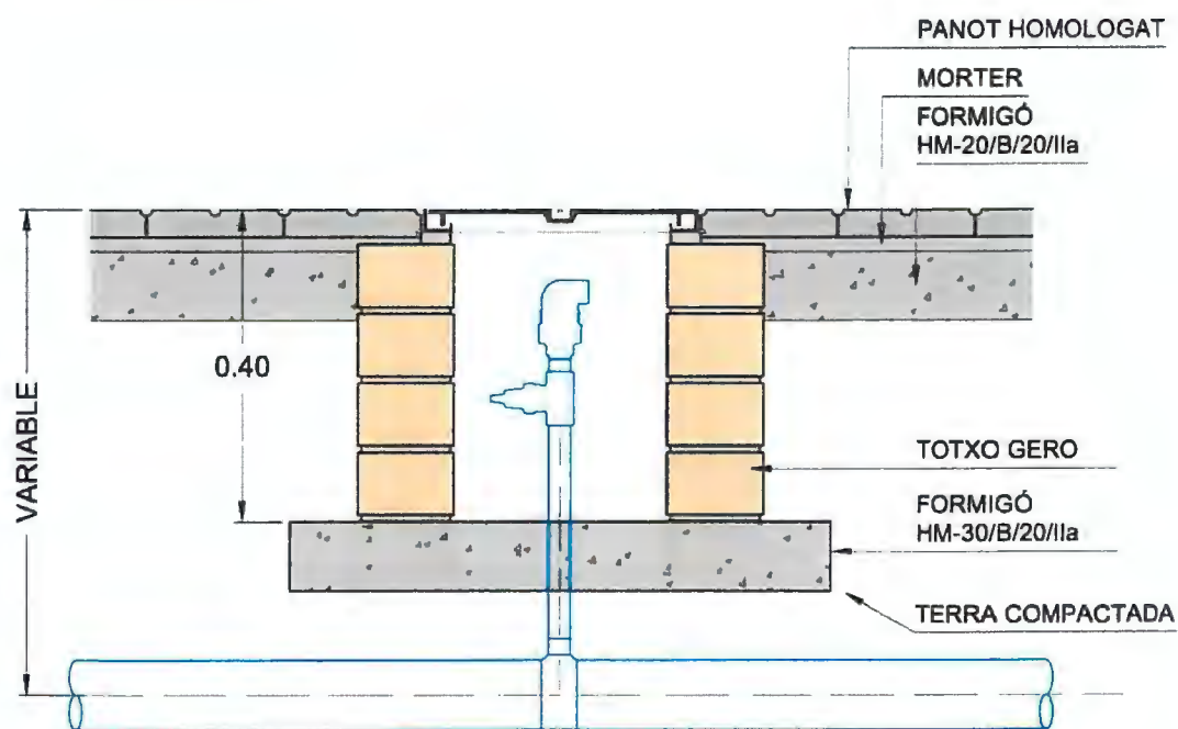
SECCIÓ
