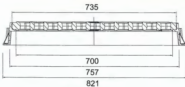
SECCIÓ B-B'
