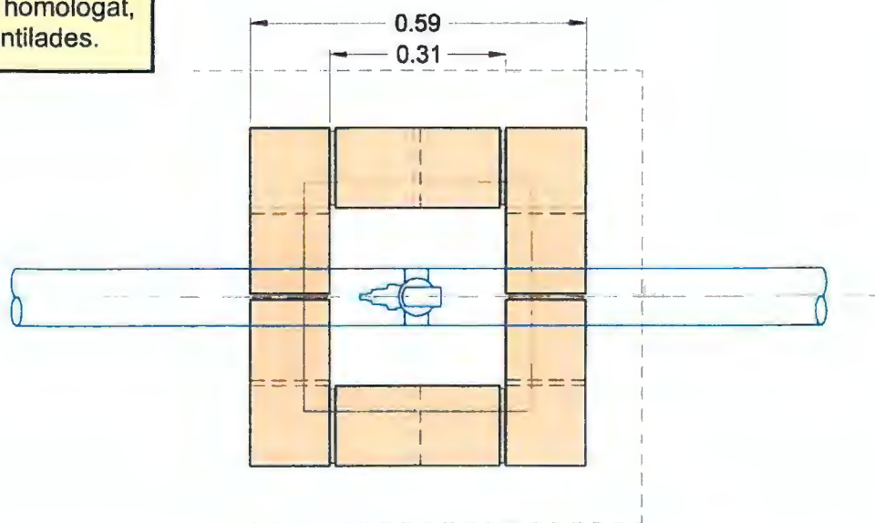
PLANTA
