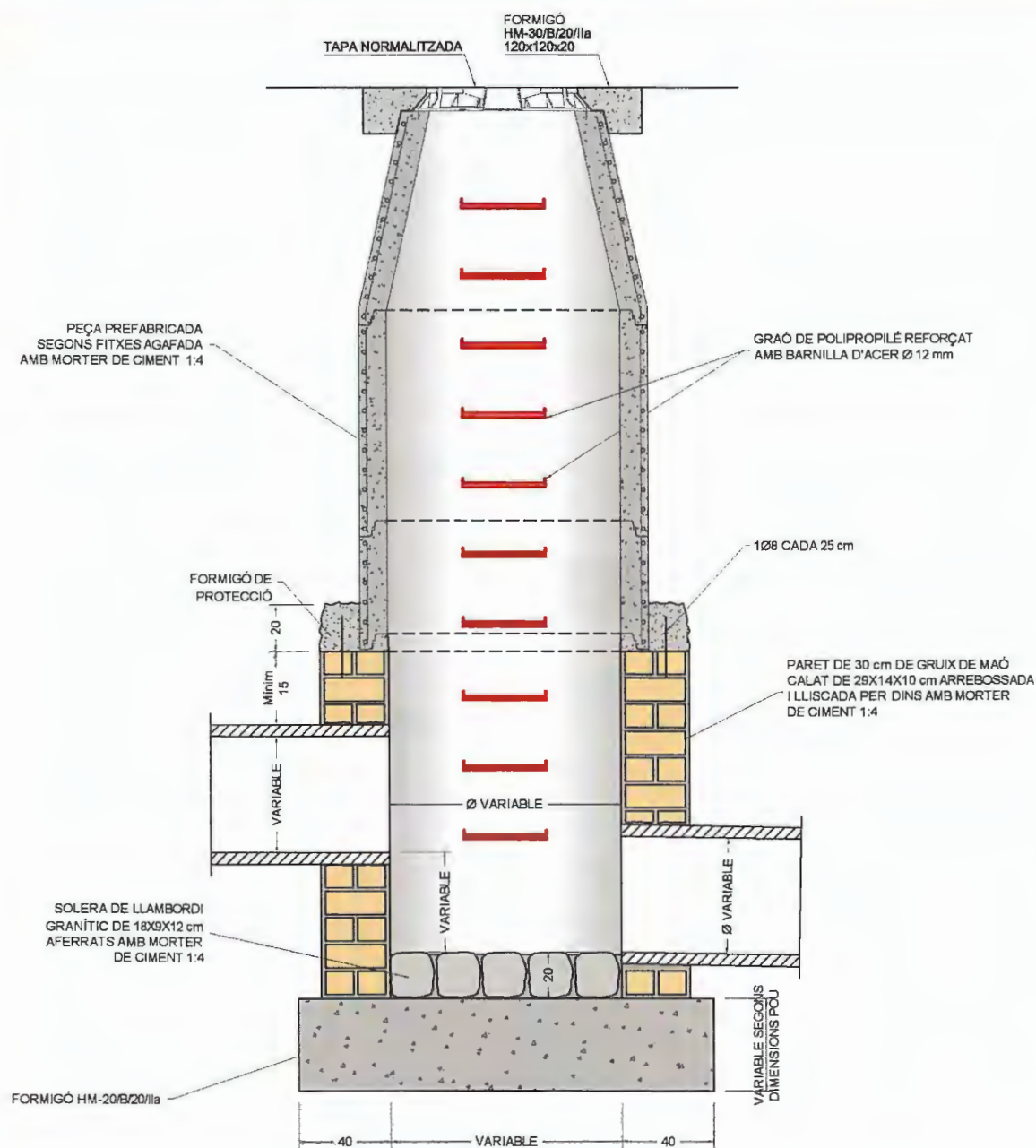
POU DE RESSALT Cotes en cm.
