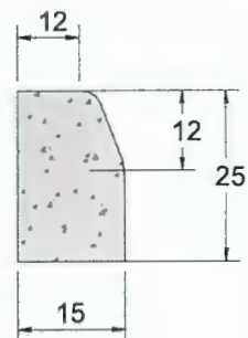
ALÇAT
