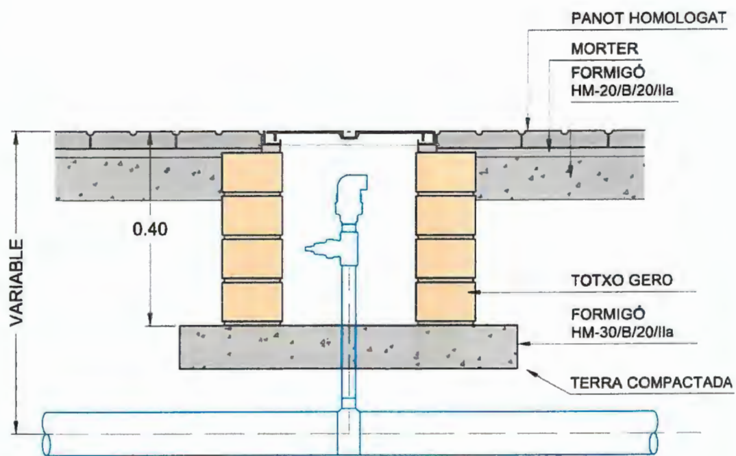
SECCIÓ
