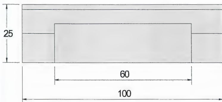
ALÇAT
