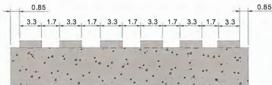
ALÇAT
