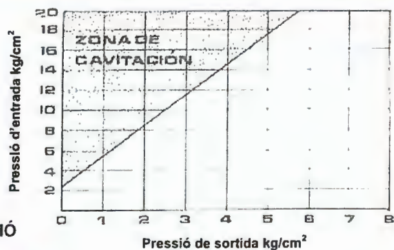
GRÀFIC DE CAVITACIÓ
