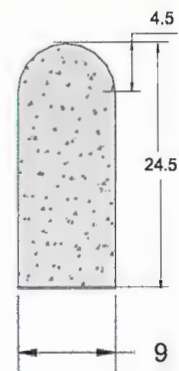
ALÇAT
