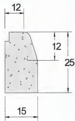
ALÇAT
