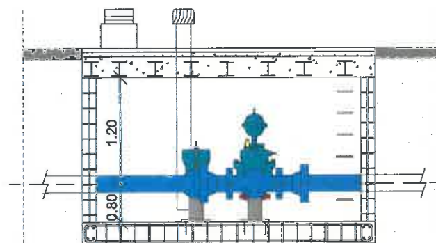
SECCIÓ A-A'
