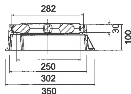
SECCIÓ A-A'
