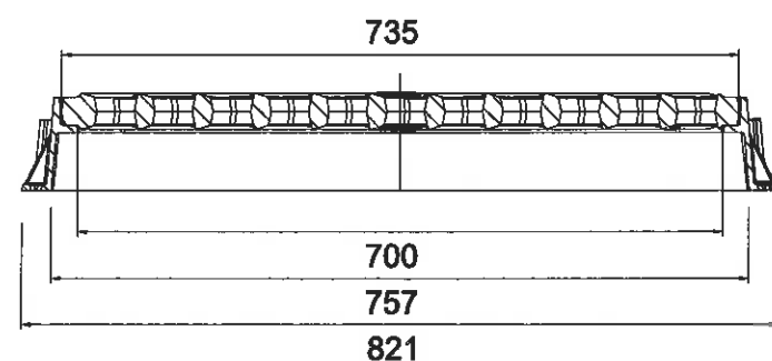
SECCIÓ B-B'
