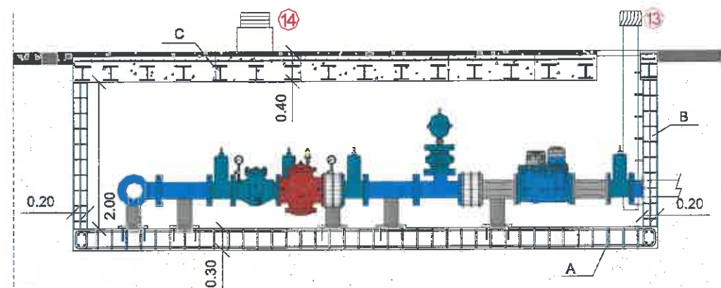
SECCIÓ B-B'
